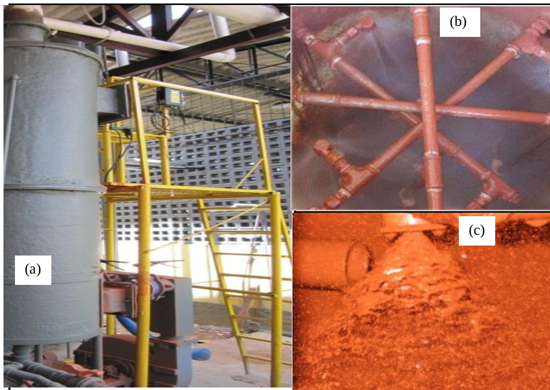
Figura 3.15 – Torre de aspersão com dez bicos centrífugos em dois níveis (a). No detalhe (b), podem ser vistos os bicos em teste com água e com suspensão de RB (c).
