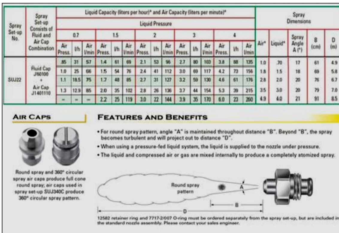
Figura 3.10 – Bico gerador de névoa de água com uso de ar comprimido, selecionado entre 90000 itens para atender os requisitos de forma da pluma, vazão de água e ar.
