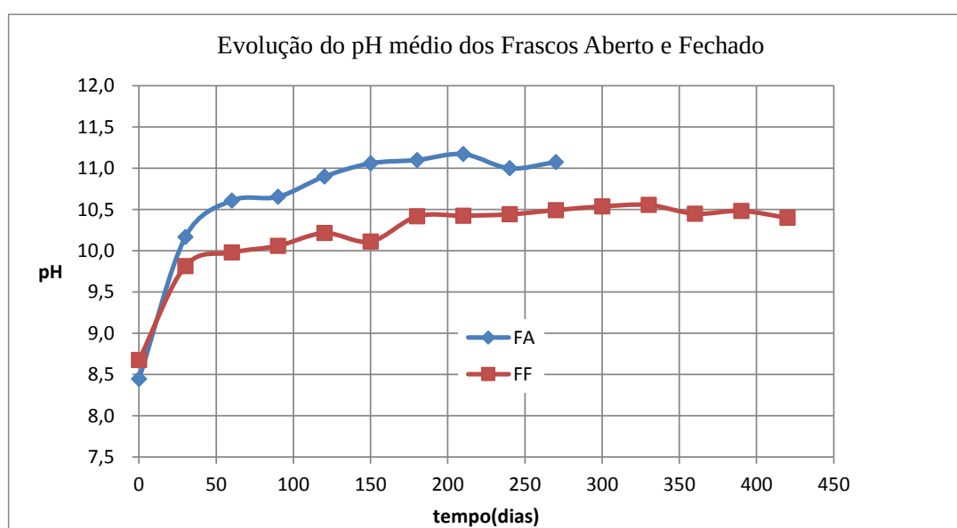
Figura 4.14 - Evolução do pH médio após os experimentos com RB em frascos tampados e abertos.
