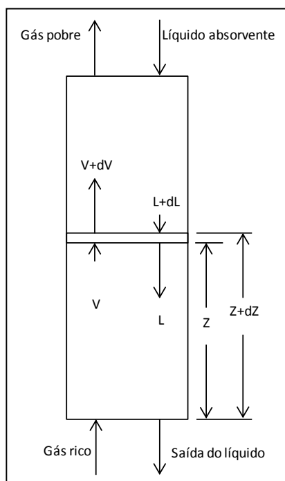
Figura 2.19 – Representação esquemática de uma torre de recheios. Fonte: BROWN G.G., (1965)
