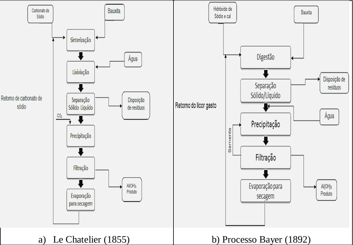
Figura 2.1: Fluxograma dos processos históricos de fabricação de alumina. Fonte: FRANÇA et al. (2007) com modificações.
