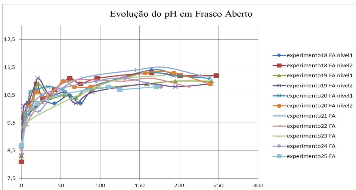
Figura 4.13 – Gráfico da evolução do pH das amostra de RB carbonatado conservadas em frasco aberto.
