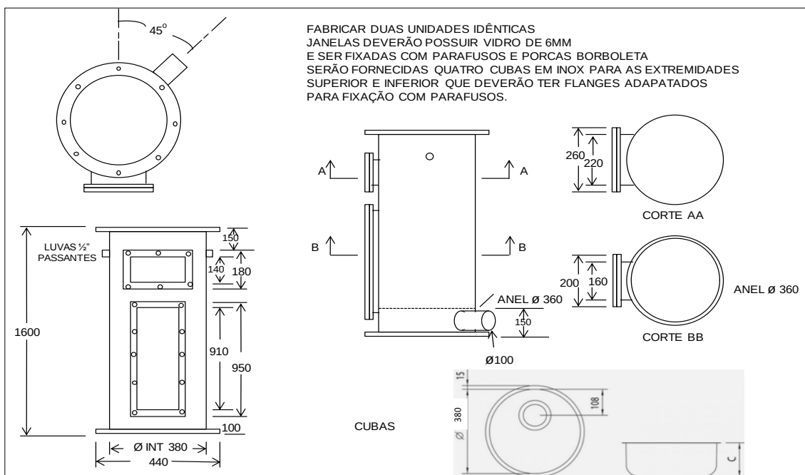
Figura 3.16 – Projeto das torres de recheio que foram fabricadas em aço inoxidável.
