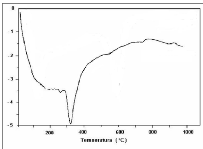
Figura 3.3 - Curva da análise térmica diferencial do RB da Alunorte. Fonte: HILDEBRANDO, 1998
