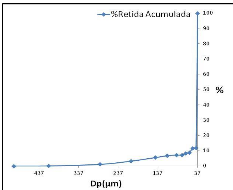
Figura 3.2 – Histograma da análise granulométrica do RB da Alunorte. Fonte: LEMOS,, 2008 (modificado).
