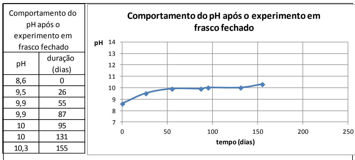
Figura 4.5 – Monitoramento da evolução do pH após o experimento 24 em frasco fechado.
