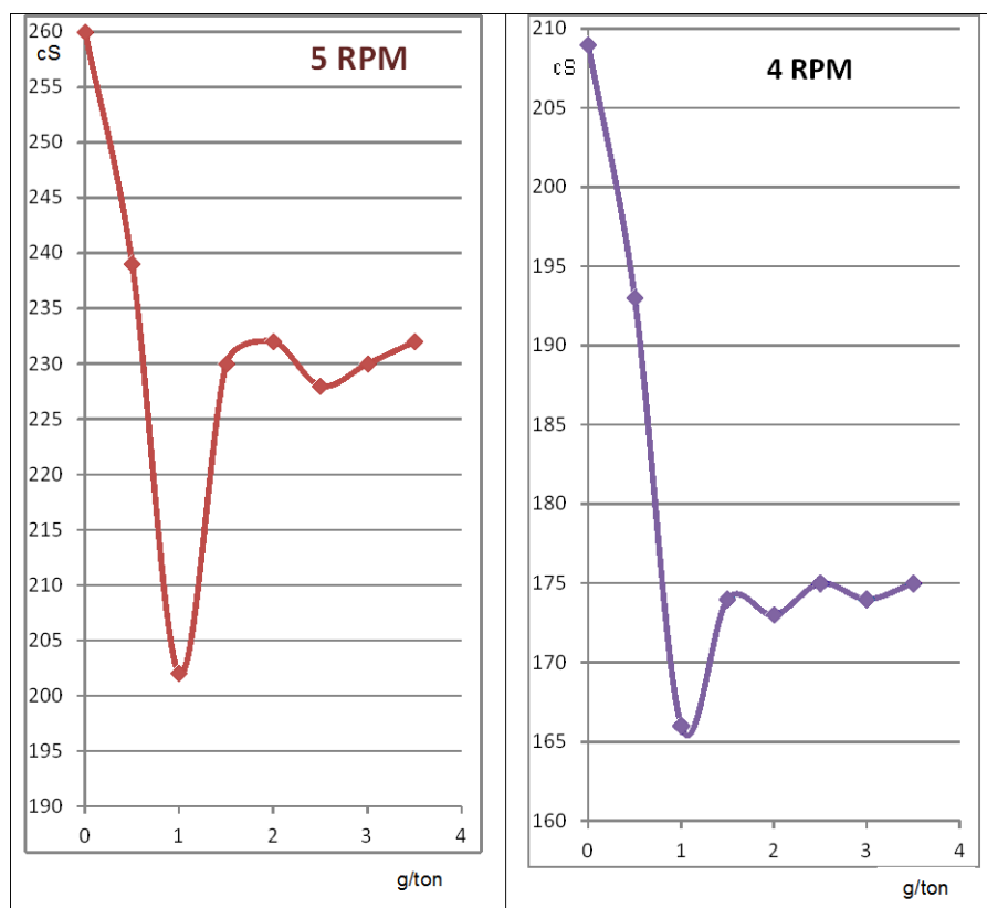
Figura 4.17 – Variação da viscosidade em função do teor de defloculante.
