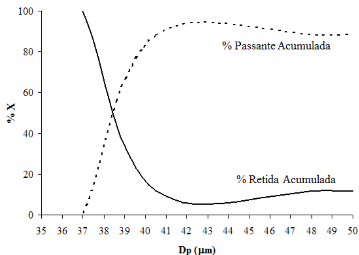
Figura 3.1 - Análise granulométrica do RB da Alunorte. Fonte: LEMOS, 2008.
