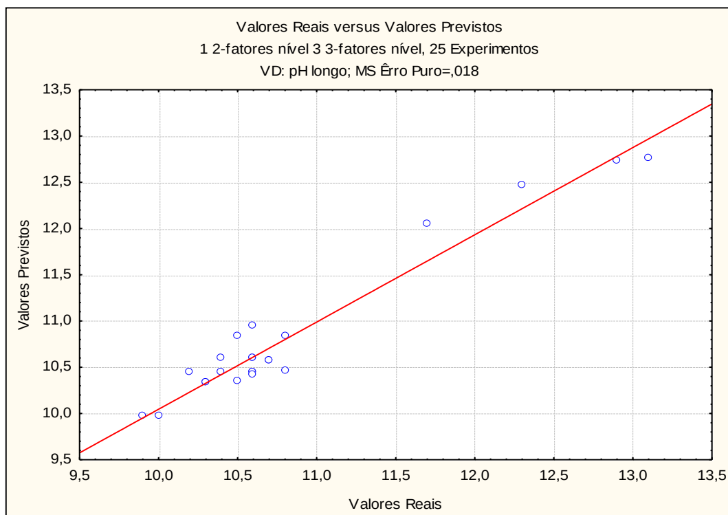
Figura 4.23 – Gráfico dos valores previstos versus reais utilizando a equação de simulação.
