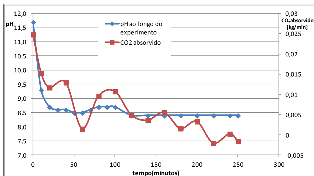
Figura 4.6 – Evolução do pH e do fluxo de absorção de CO 2 no experimento 22.
