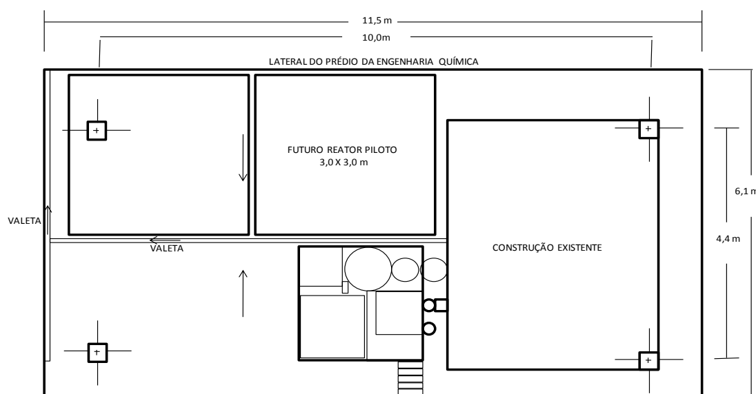
Figura 3.6 – Planta baixa do galpão com 70 m 2 projetado e construído para a realização dos experimentos. Fonte: autor.
