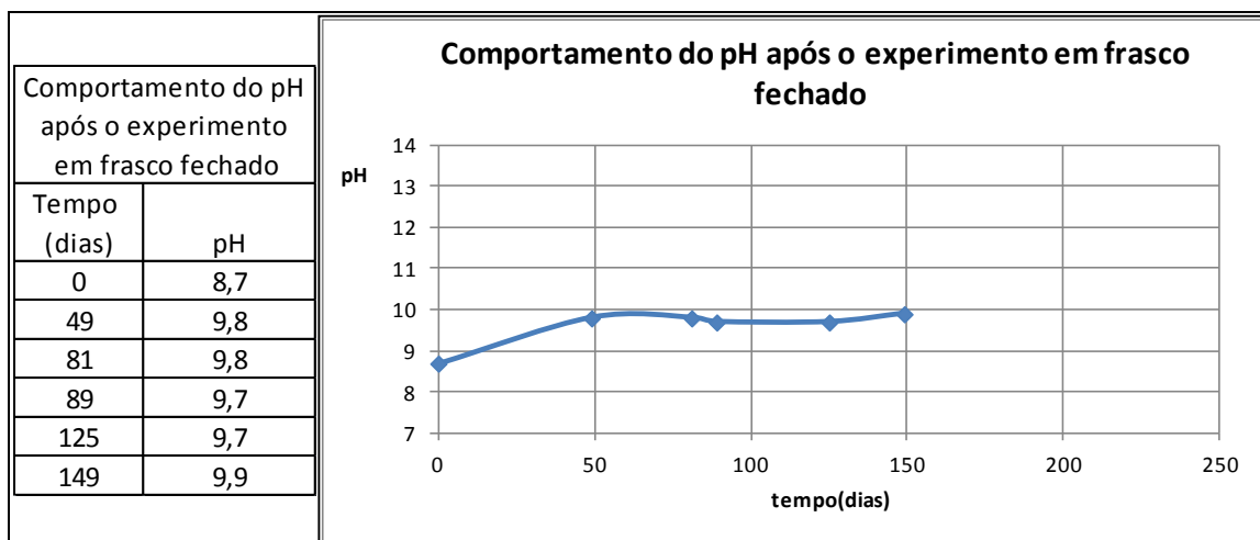
Figura 4.2 – Monitoramento da evolução do pH após o experimento 25 em frasco fechado.
