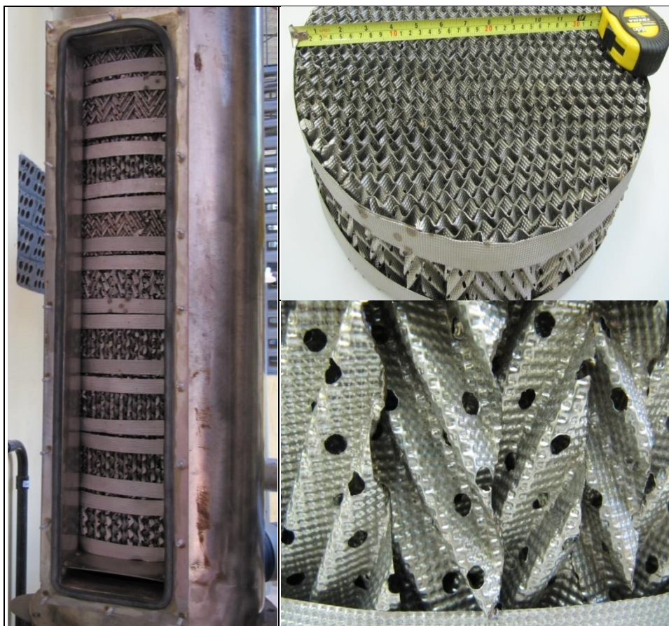
Figura 3.19 – Torre de recheio preenchida com recheio estruturado de alto desempenho, nos detalhes um módulo do recheio estruturado e as lâminas que o compõem e geram uma hidrodinâmica mais eficiente.
