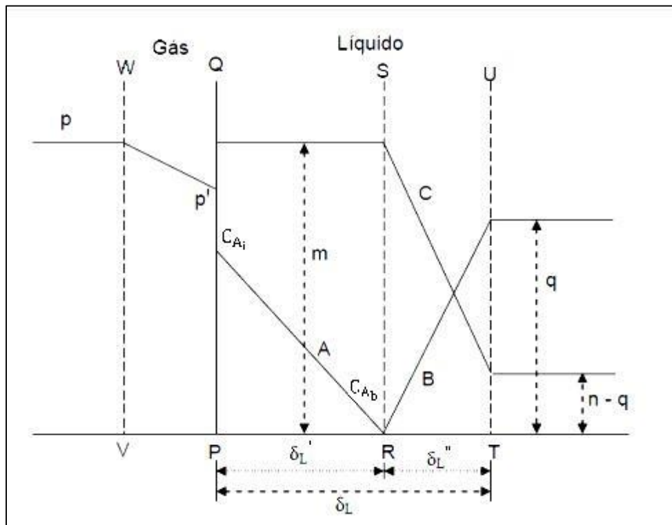
Figura 2.18 – Concentrações em um processo com reação química conforme modelo do filme duplo. Fonte: SHERWOOD e PIGFORD (1975).
