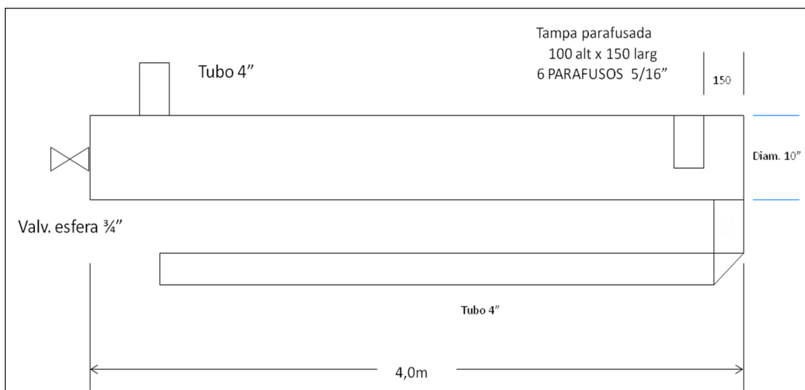
Figura 3.8 – Projeto do trocador de calor tubular de contato direto em contracorrente.
