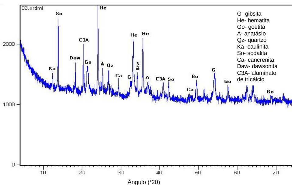
Figura 4.15 - Difração de raios X da amostra de RB não reagido da Alunorte. Fonte: autor.
