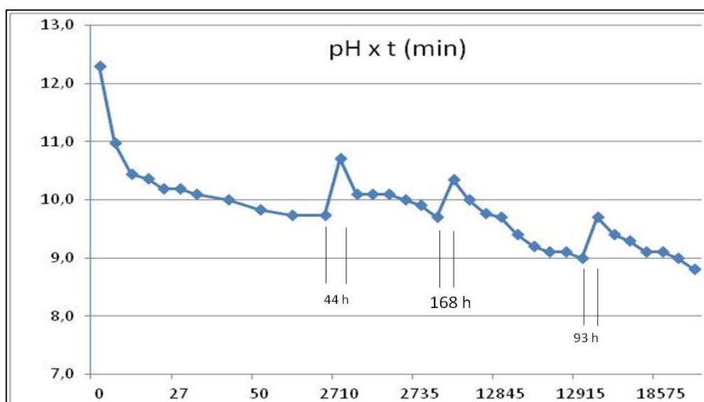
Figura 4.7 – Gráfico da evolução do pH durante o experimento de número 2.
