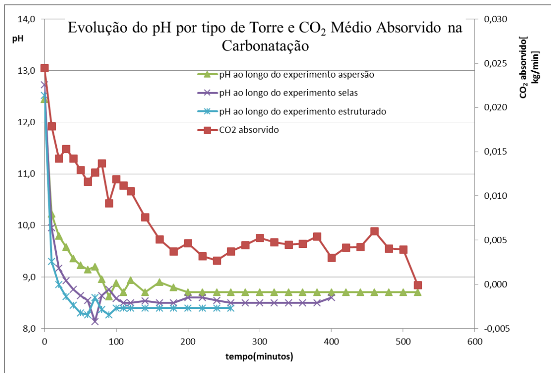
Figura 4.11 – Gráfico comparativo das médias de evolução do pH por tipo de torre e CO 2 médio absorvido.
