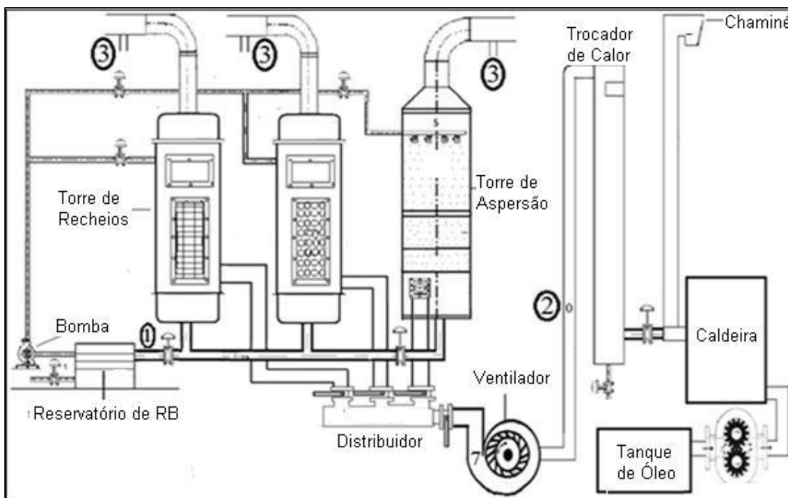
Figura 3.35 – Pontos de medição mostrados no desenho esquemático do processo.
