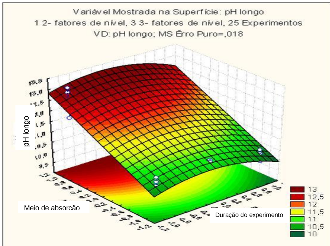
Figura 4.20 – Gráfico mostrando a superfície de resposta do pH longo.
