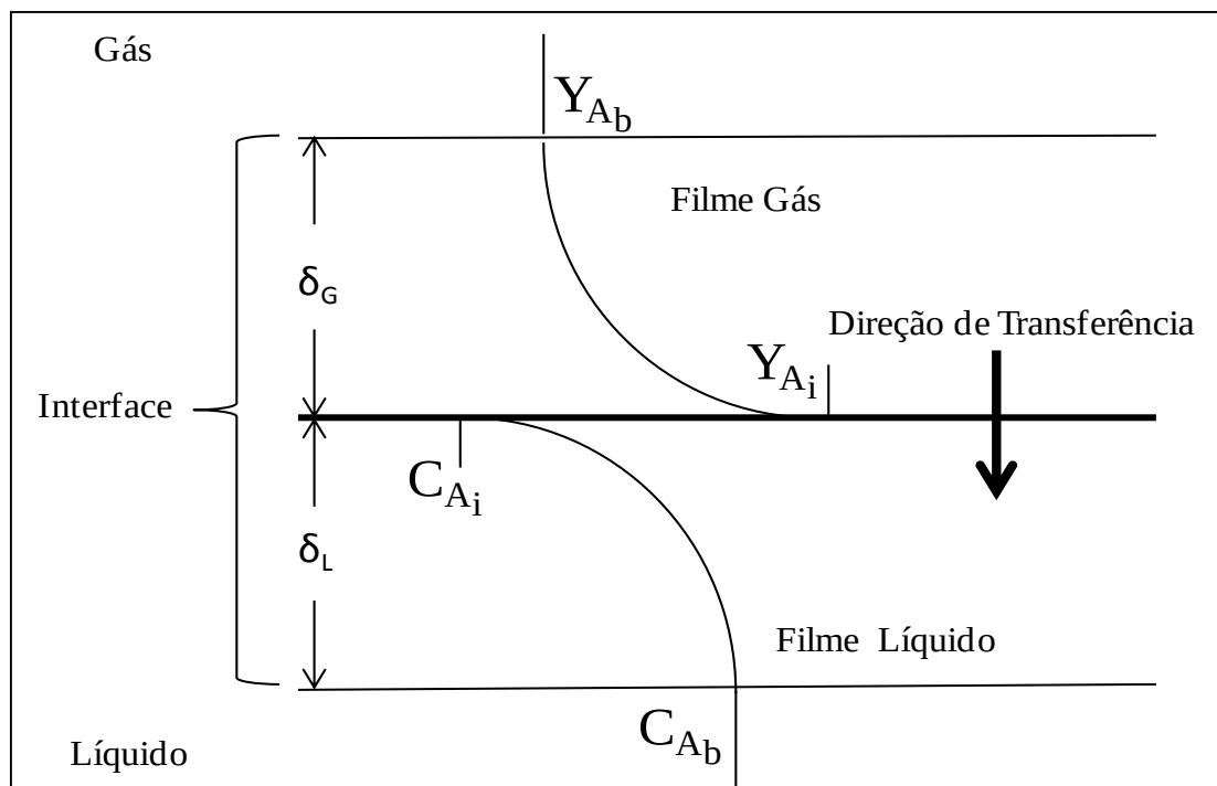
Figura 2.17 – Modelo de dois filmes Fonte: SHERWOOD e PIGFORD (1975)
