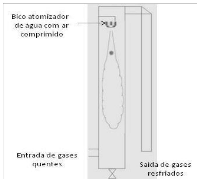
Figura 3.12 – Desenho esquemático do trocador de calor de contato direto em contracorrente.
