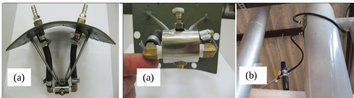
Figura 3.11 – Bico gerador de névoa (a) montado no topo do trocador e conectado ao regulador de pressão de ar (b) e a alimentação de água.
