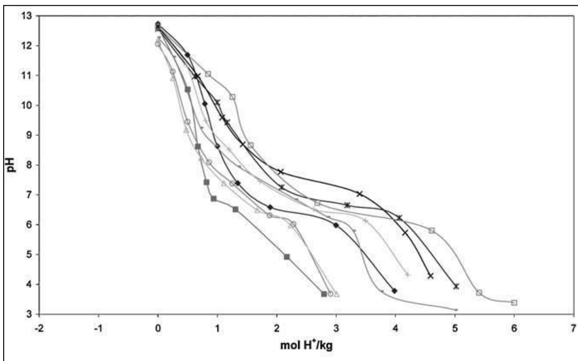
Figura 2.13 - Curvas de capacidade de neutralização ácida do RB de nove diferentes refinarias da Austrália. Fonte: CARTER, C., VAN DER SLOOT, H. et al. (2008).
