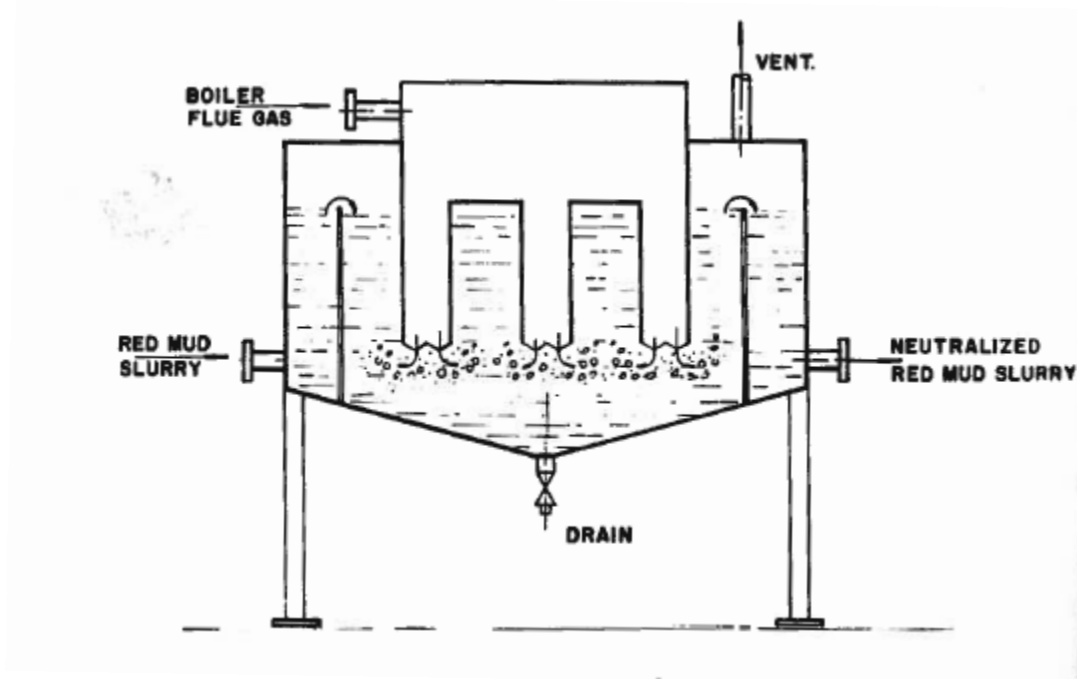
Figura 2.22 – Primeiro experimento de redução da reatividade de RB conforme ilustração original. Fonte: VERSIANI, 1983.
