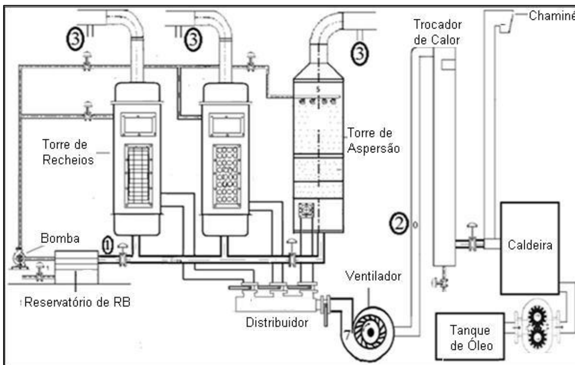
Figura 3.5 – Desenho esquemático dos equipamentos com a indicação dos pontos de coleta de amostras.
