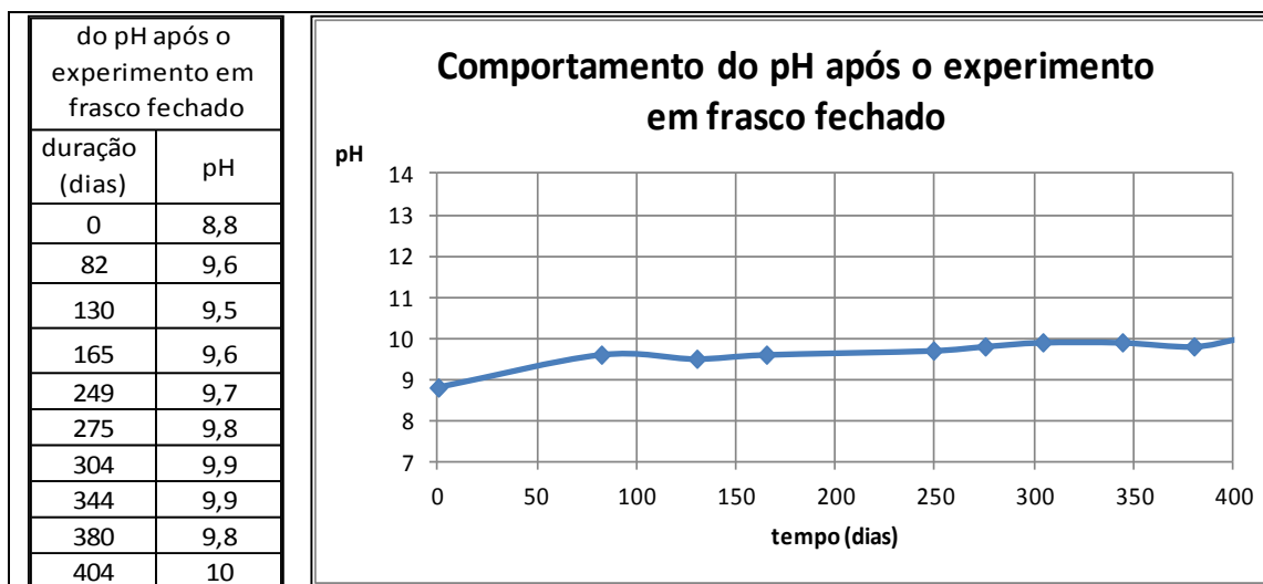
Figura 4.8 – Evolução do pH de longo prazo do experimento 2 em frasco fechado.
