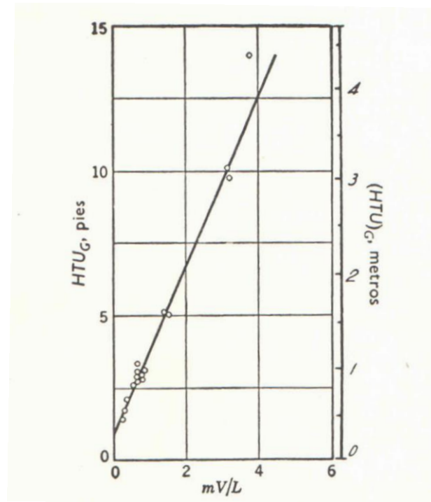
Figura 2.20 – Altura de unidade de transferência ( HTU_G ) em função de mV/L para absorção de SO_2 por H_2O utilizando anéis de 3 polegadas, com espiral interior. Fonte: BROWN, G.G. (1965).
