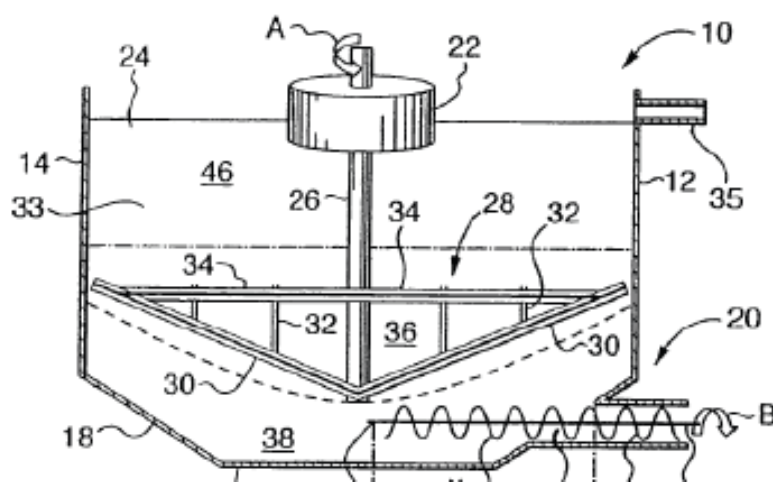
Figura 2.5 – Desenho esquemático da patente de espessador de última geração pertencente a empresa Rio Tinto. Fonte: PELOQUIN et al. , patente US7,473,376 (2009).
