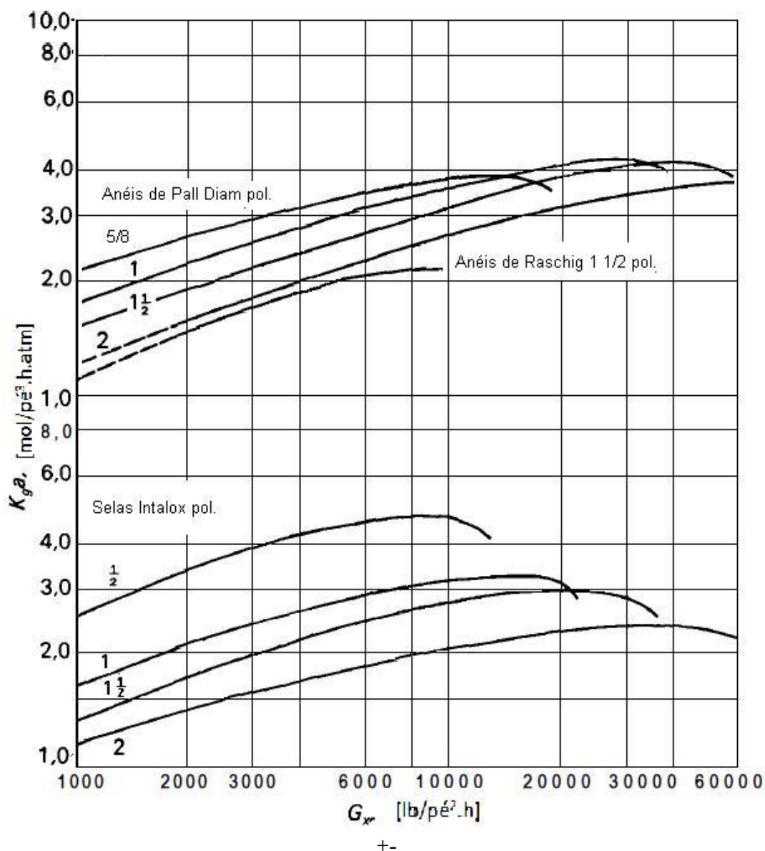
Figura 2.21- Coeficientes de transferência de massa para absorção de \text{CO}_2 em solução de NaOH 4%-p utilizando diferentes recheios. Fonte: McCABE (1985).
