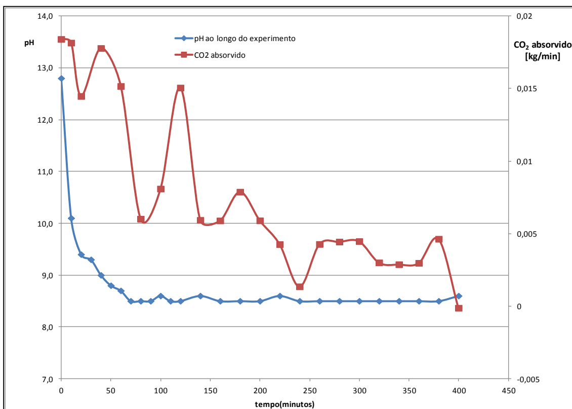
Figura 4.4 - pH e a vazão de massa de CO 2 absorvida durante o experimento 24.
