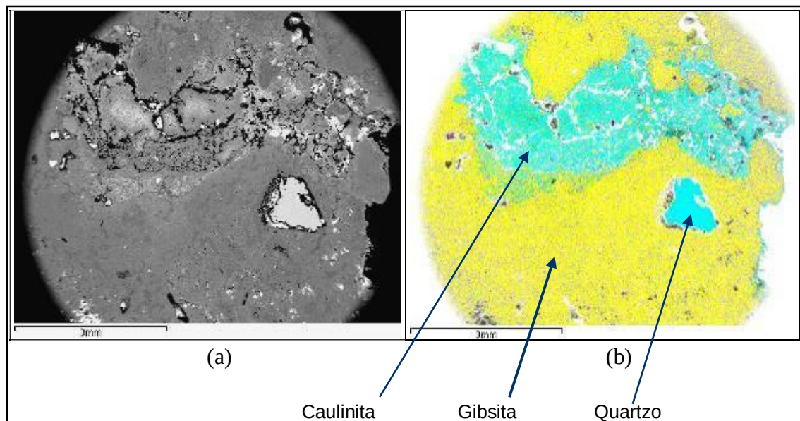
Figura 2.2 – (a) Micrografia da bauxita de Paragominas (b) Mapeamento da micrografia. Fonte: FRANÇA et al. (2007).
