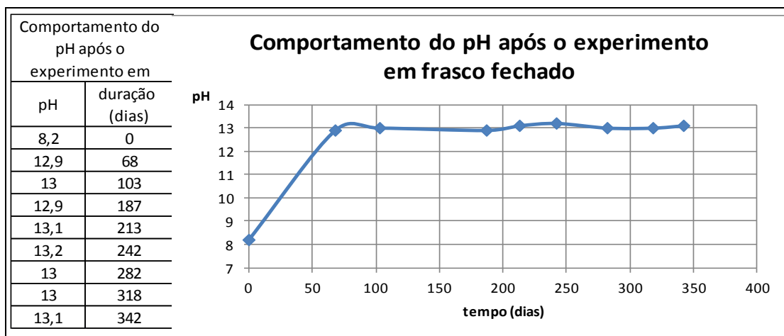
Figura 4.10 – Evolução do pH de estabilização em frasco fechado do experimento 11.
