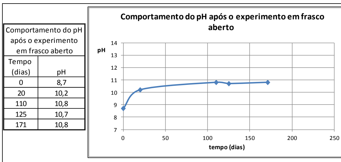
Figura 4.3 – Monitoramento da evolução do pH após o experimento 25 em frasco aberto.
