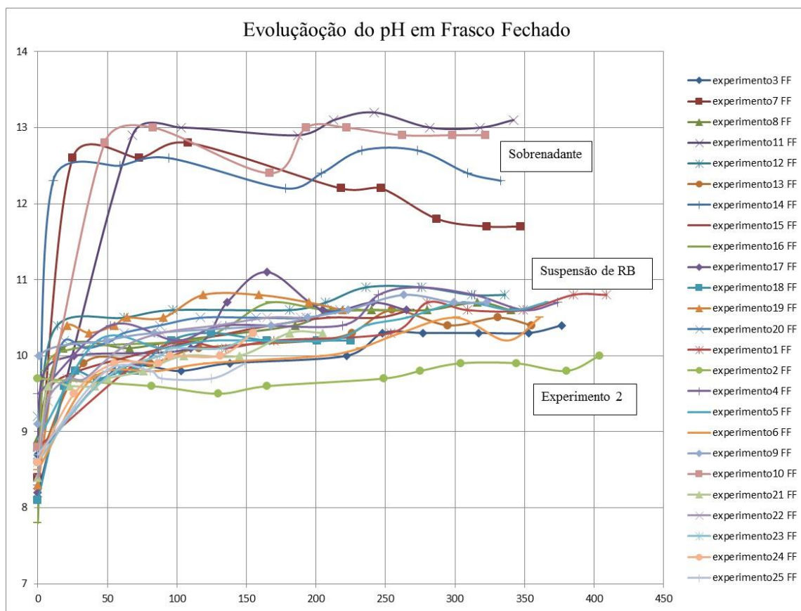
Figura 4.12 – Gráfico da evolução do pH das amostras de RB carbonatado conservadas em frasco fechado.
