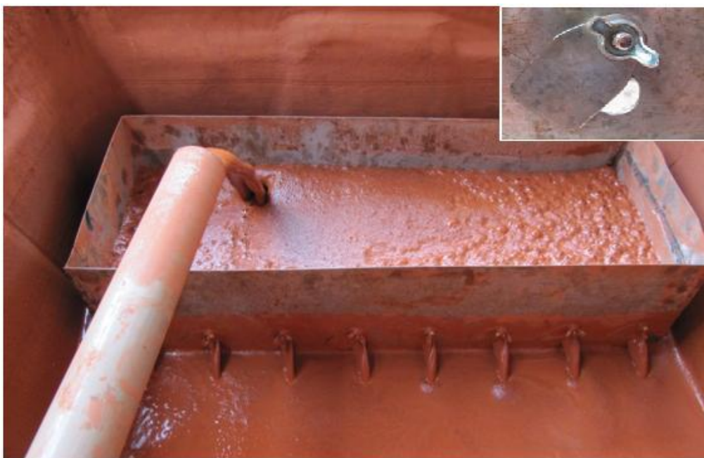
Figura 3.26 – Vista da caixa de retorno com dez saídas ajustáveis destinadas a reduzir a turbulência no retorno do RB.
