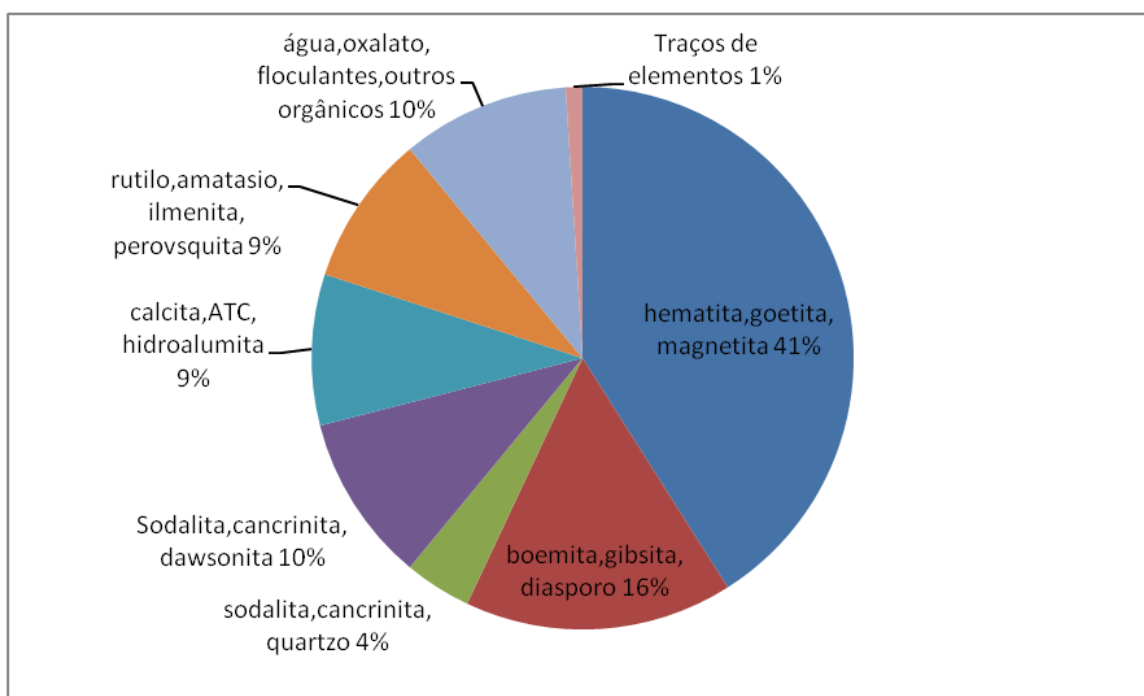
Figura 2.12 – Visão mineralógica da composição do RB. Fonte GRÄFE et al. (2009)
