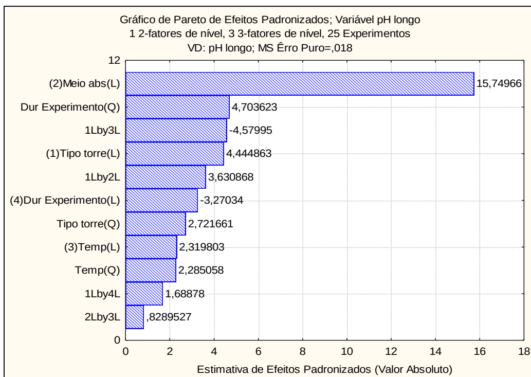
Figura 4.19 – Gráfico de Pareto mostrando o impacto das variáveis e suas interações.
