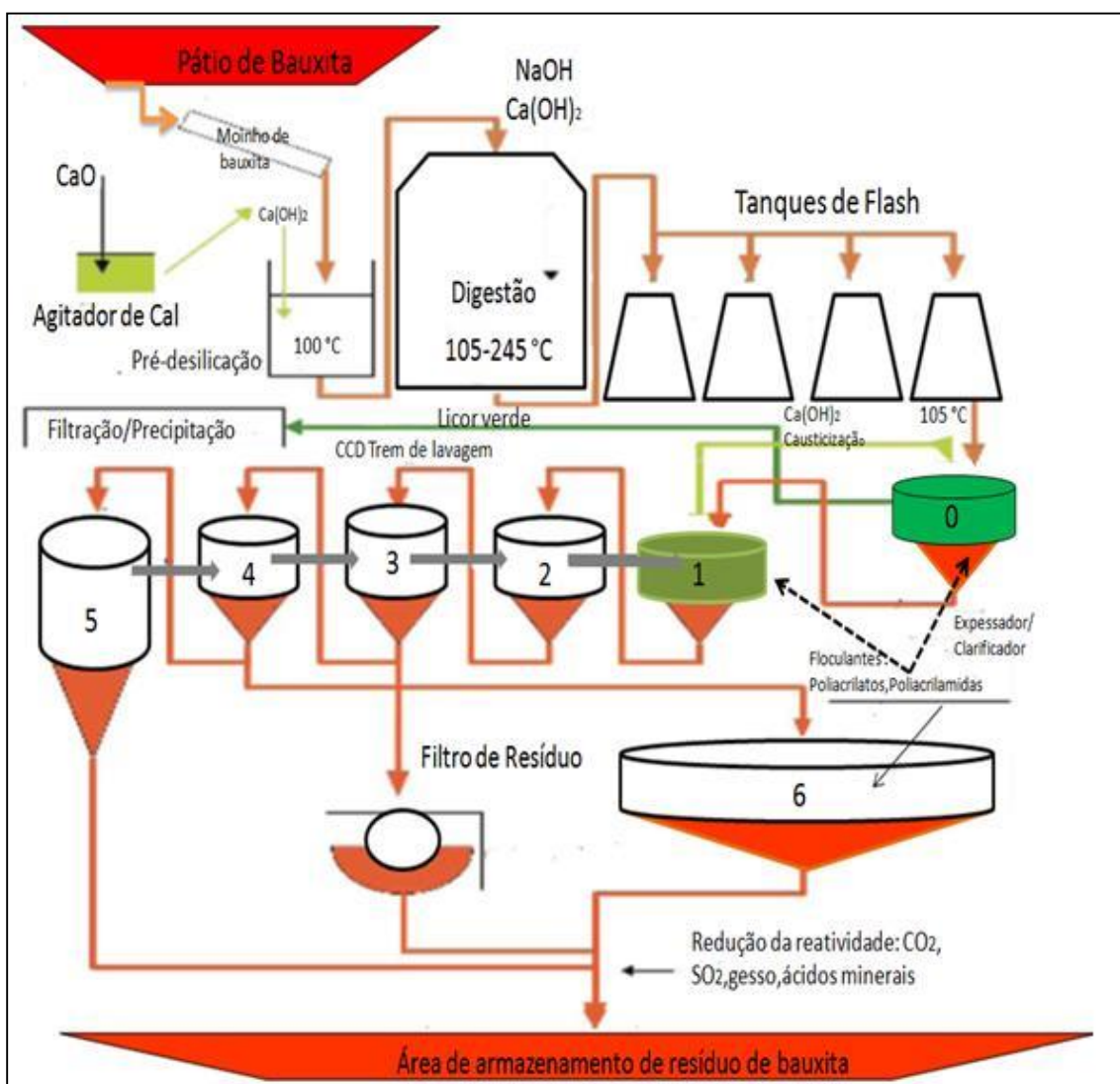
Figura 2.10 - Fluxograma de formação do RB indicando locais de entrada de NaOH, \text{Ca(OH)}_2 e floculante. As setas cinza indicam a direção da água de lavagem em contracorrente do fluxo de RB. Adotado com modificações a partir de WHITTINGTON (1996).
