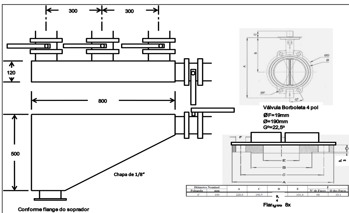
Figura 3.13 – Projeto do distribuidor de gases dotado de quatro válvulas tipo borboleta.
